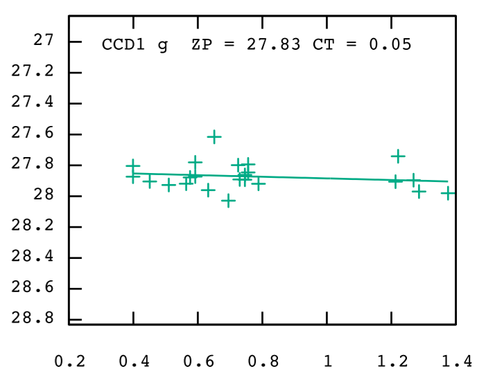
(g-i)
