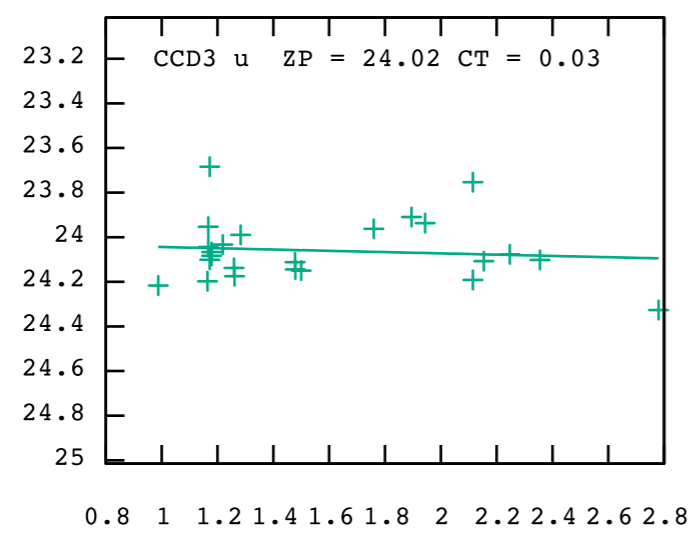
(u-g)
