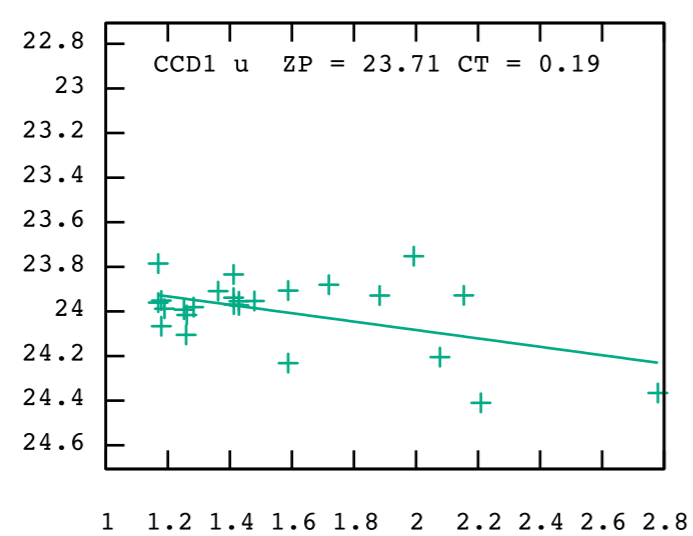
(u-g)
