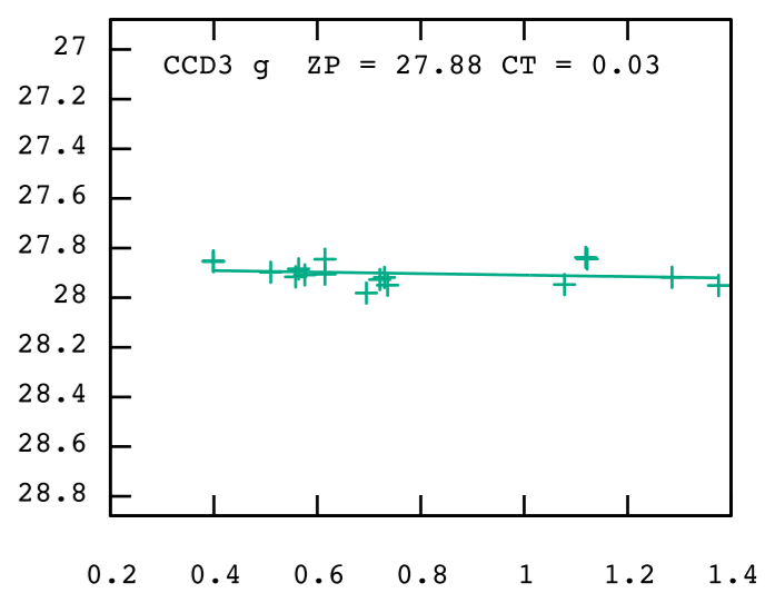
(g-i)
